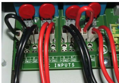
Fig. 12A - Collegamenti presenti su una unità uscita di fabbrica
