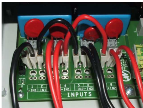
Connessione parallelo dei due canali
