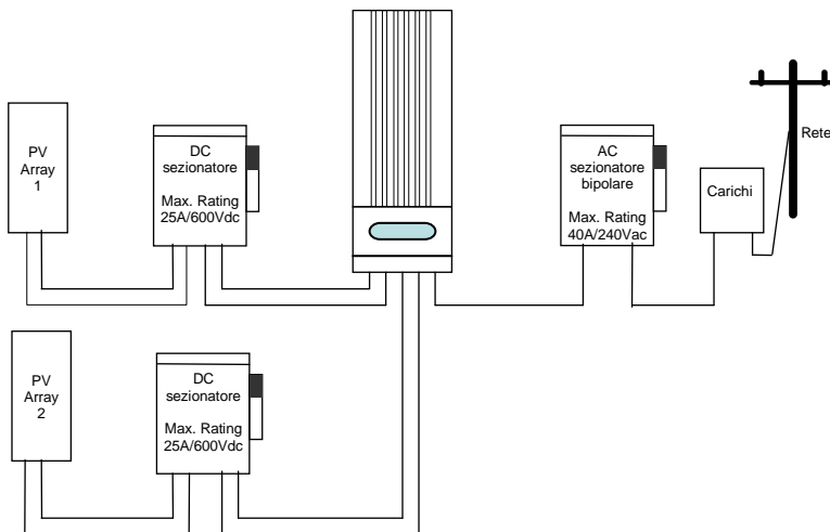
Fig. 9 - Diagramma di collegamento
