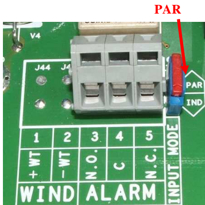
Configurazione dell' Inverter in modalità "parallelo"
