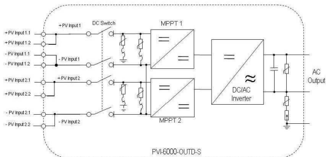
Fig. 3B - Schema funzionale inverter con DC switch integrato
