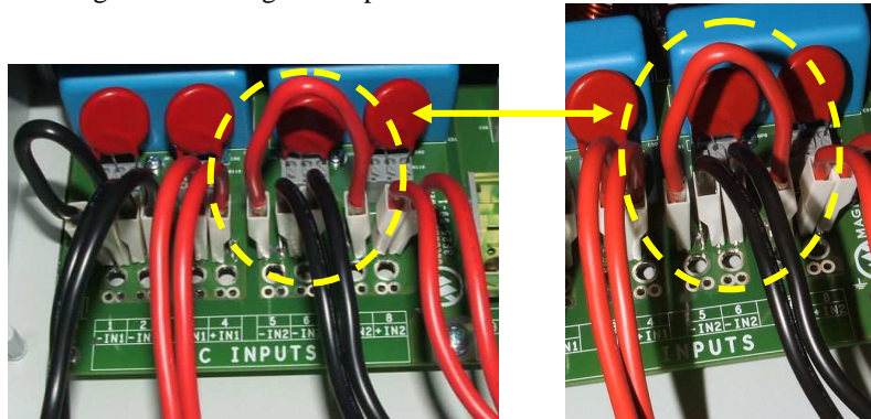
Fig. 12A - Collegamenti presenti su una unità uscita di fabbrica
