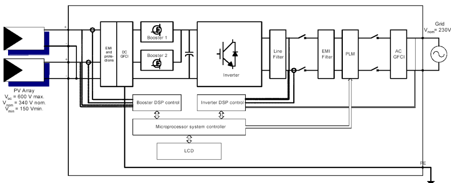
Fig. 4 - Diagramma a blocchi AURORA
