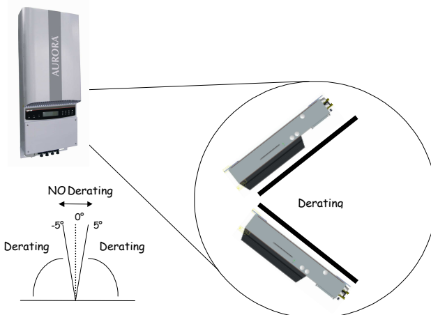
Fig. 8 - Montaggio in posizione inclinata
