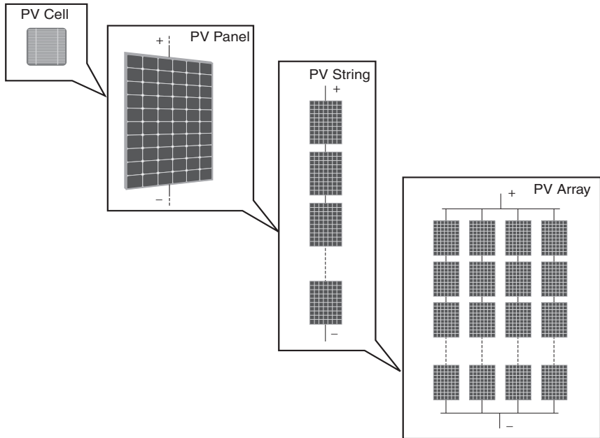
Fig. 2 - Composizione Array
