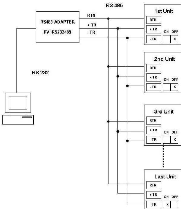
Fig. 25 - Connessione multipla daisy-chain
