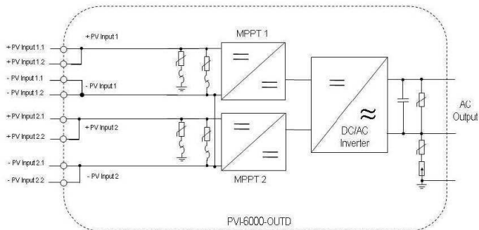
Fig. 3A - Schema funzionale inverter senza DC switch integrato
