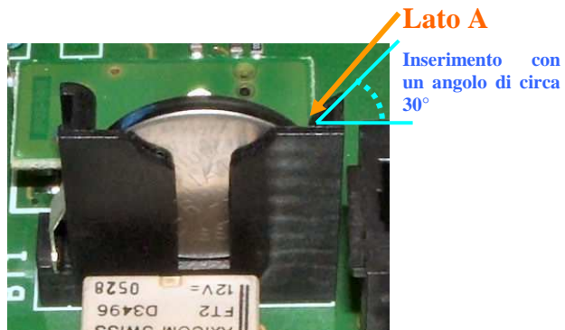
Fig. 15 - Batteria all'interno di Aurora
