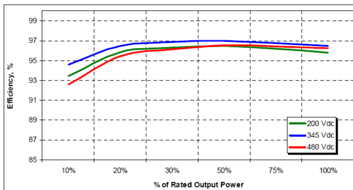
Fig.29 curve di efficienza
