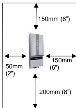
Fig. 5 - Luogo di installazione - Spazio minimo intorno a AURORA
