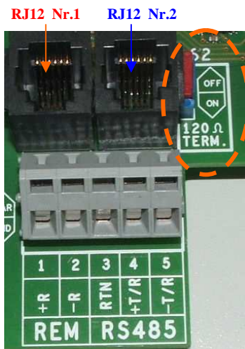
Fig. 24 - Morsetti di collegamento alla linea seriale RS-485 e interruttore S2
