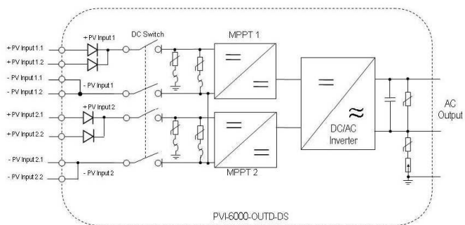
Fig. 3C - Schema funzionale inverter con DC switch e diodi di protezione integrati.
